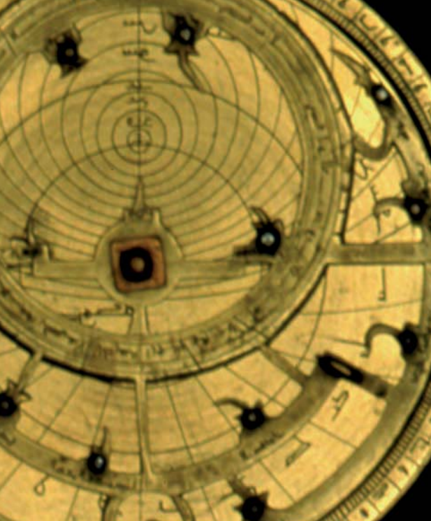
Astrolabe yéménite, XV e siècle © IMA/Savel L'astrolabe planisphérique permet de calculer la hauteur des étoiles et leurs mouvements pour une latitude donnée. Grâce à cet outil complexe mais transportable, les voyageurs pouvaient notamment se repérer la nuit.
