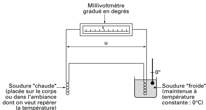
Fig. 3. Utilisation d'un thermocouple.
