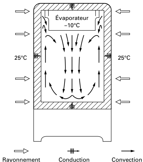
Fig. 1. Transmission de la chaleur à travers les parois d'un réfrigérateur. Association des trois modes de transmission.
