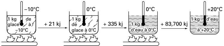
Comparaison de la chaleur latente et de la chaleur sensible
