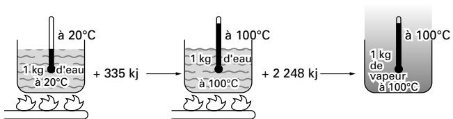
Chaleur sensible et chaleur latente de vaporisation de l'eau
