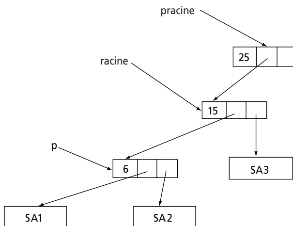
Figure 88 Arbre avant réorganisation GG.
