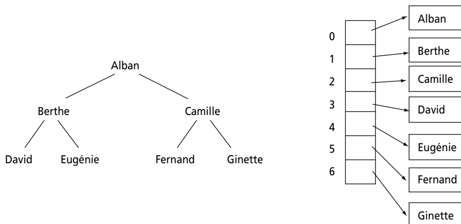
Figure 76 Mémoire d'un arbre binaire complet.
