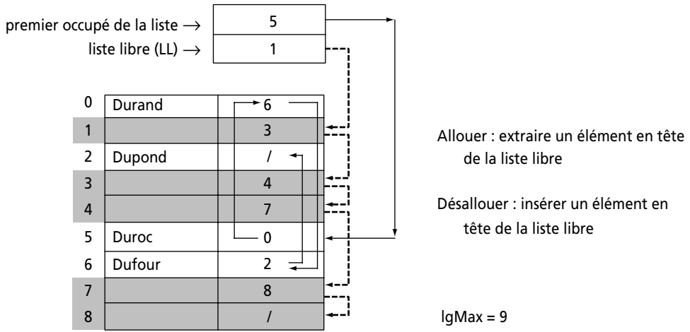
Figure 43 Gestion d'espace mémoire avec une liste libre.
