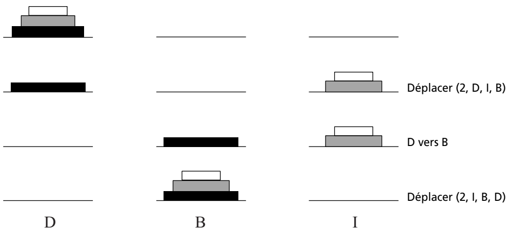
Figure 6 Tours de Hanoi : principe.
