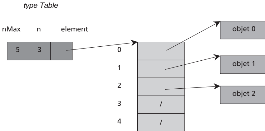
Figure 118 Le type Table (les pointeurs des objets sont consécutifs).
