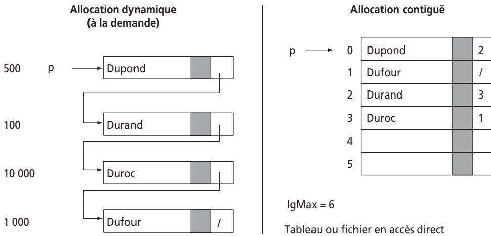
Figure 20 Mémorisation des listes (dynamique ou contiguë).
