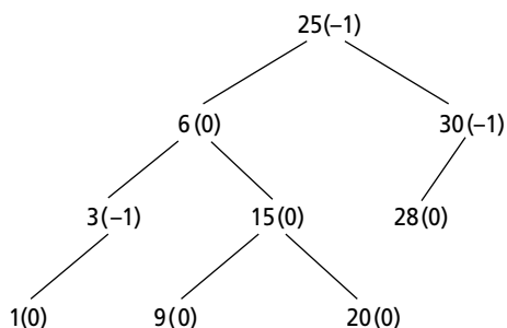
Figure 87 Arbre après rééquilibrage GG de 6 et 15.
