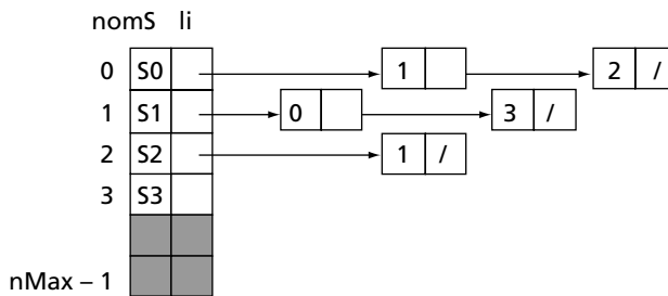
Figure 147 Mémorisation sous forme d'une table de listes d'adjacence.
