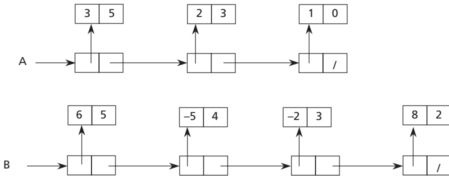
Figure 26 Mémorisation de polynômes sous forme de listes.
