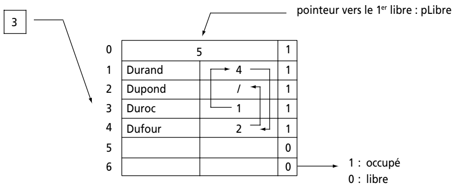
Figure 41 Gestion d'un espace mémoire (tableau ou fichier).
