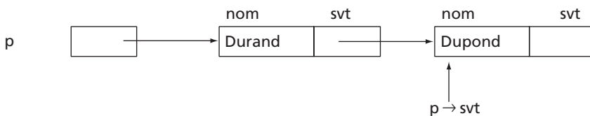
Figure 15 Le champ nom de la structure pointée par p \rightarrow svt .
