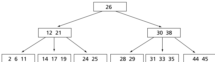
Figure 103 B-arbre d'ordre 2.
