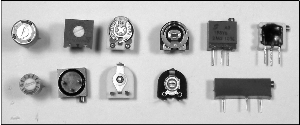
Figure 2.8.2.a - Différents types de potentiomètres ajustables pour usage grand public et professionnel. Les trois potentiomètres de droite sont de type multi-tours (10, 15 et 25 tours).
