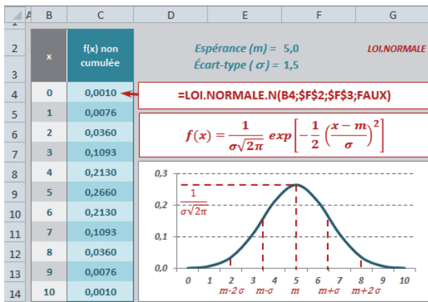
Figure 15-48 Mise en œuvre de la fonction LOI.NORMALE.N. Le graphique illustre les valeurs de la plage C4:C14, qui affiche les résultats de LOI.NORMALE.N non cumulée (fonction de densité de probabilité) pour une espérance de 5, et un écart-type de 1,5.
